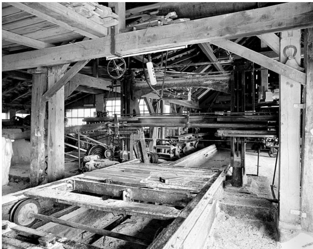
Châssis de scie horizontale monolame.
