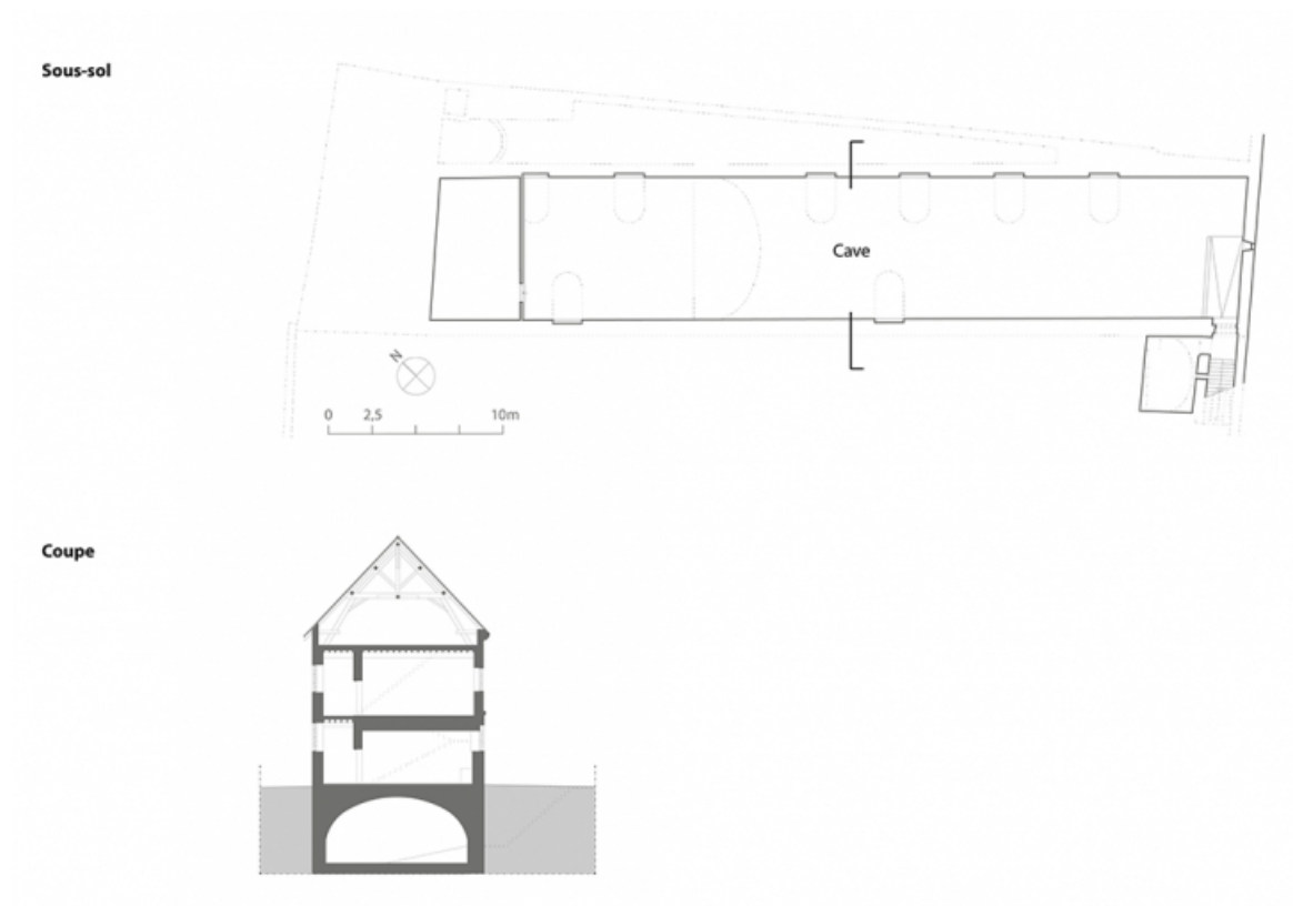
Plan du sous-sol et coupe transversale de la prison de Mâcon, échelle 1/250. 2025.
