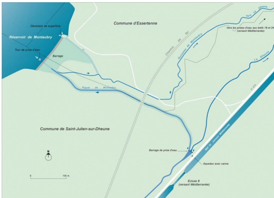
Carte schématique du barrage et de la rigole de Montaubry.
