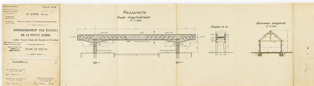
Agrandissement des écluses de la petite Saône entre Saint-Jean-de-Losne et Verdun. Ecluse de Verdun. Passerelle. 71, Bragny-sur-Saône, lieudit : près du Rompereau
