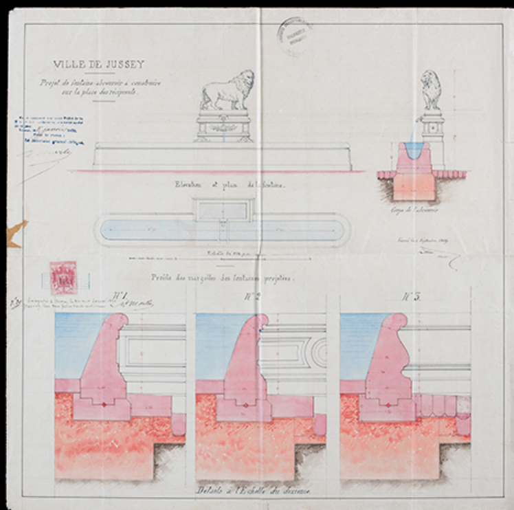
Élévation, profil, plan et coupe de la fontaine, 1869.
