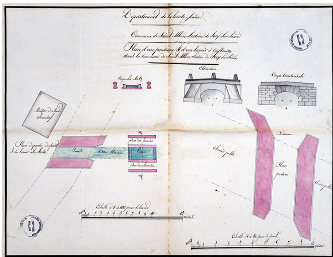
[Pambet, Marc]. Plan d'un pontceau et d'un abreuvoir à construire dans la commune de Saint-Albin section de Scey-sur-Saône. [1822].
