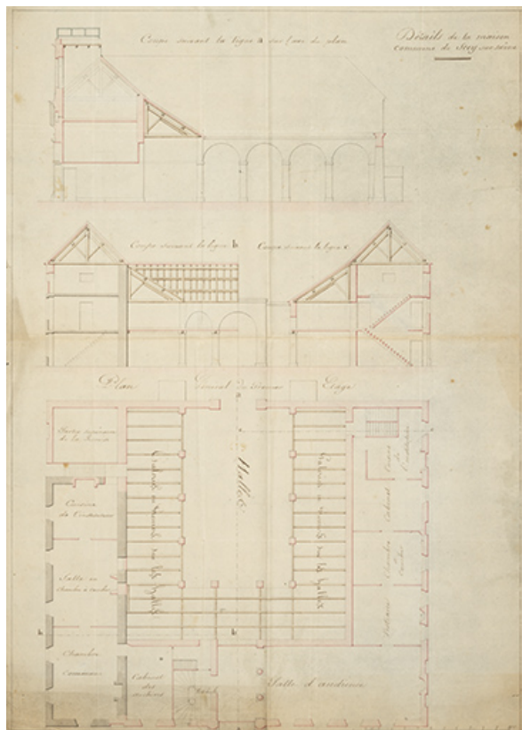
Duret. Détails de la maison commune de Scey-sur-Saône. Coupe. Plan général du premier étage. [1831].
