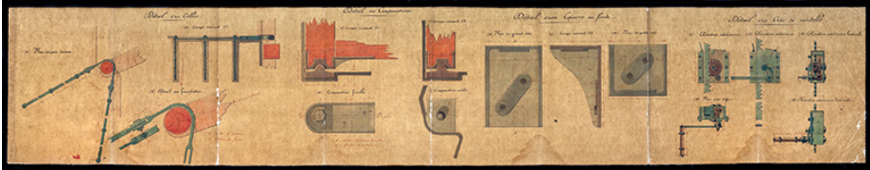
Construction du barrage mobile et de la seconde porte de garde de St-Albin - Détail des fourures de la porte de garde (1874). 70, Rupt-sur-Saône
