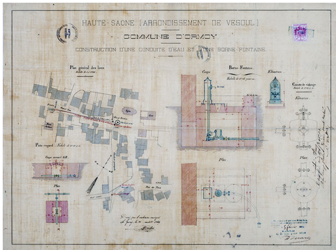
Construction d'une borne-fontaine et d'une conduite d'eau (1869).
