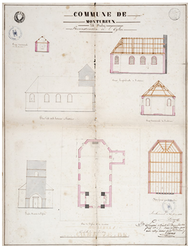
Projet de reconstruction de l'église (1838).
