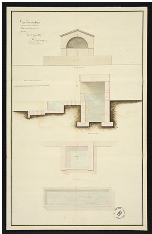
Plan d'une fontaine à construire, rue Saint-Nicolas (1829). 70, Pont-du-Bois
