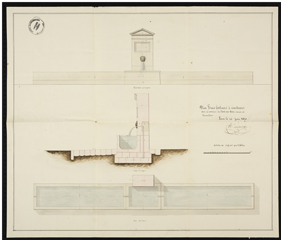
Plan d'une fontaine à construire (1829).
