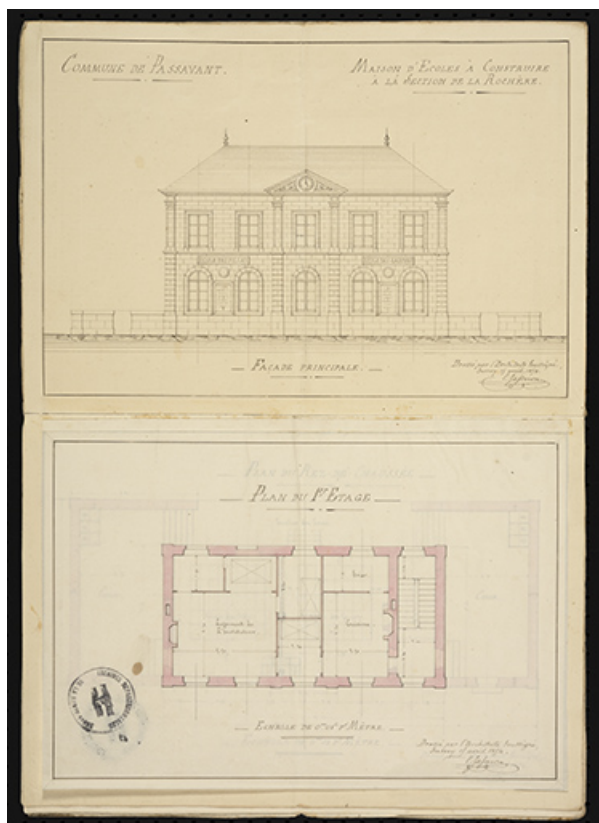
Projet de construction de l'école de la Rochère en 1854. 70, Passavant-la-Rochère, 1 place Dieu, lieudit : la Rochère
