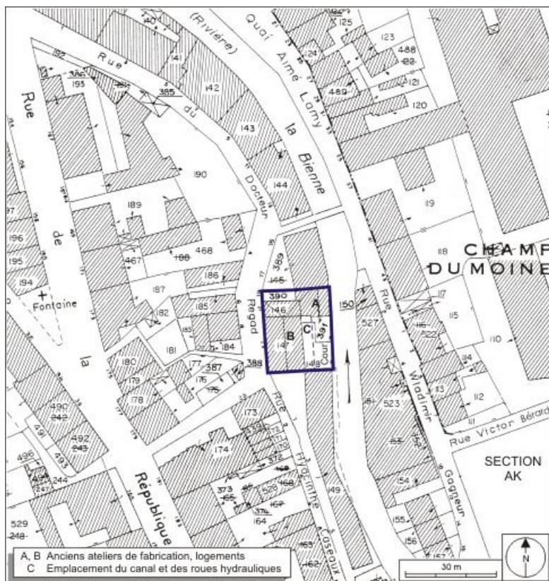
Plan-masse et de situation. Extrait du plan cadastral, 1980, section AI, échelle 1:1000. 39, Morez, 19 à 23 rue du Docteur Regad
