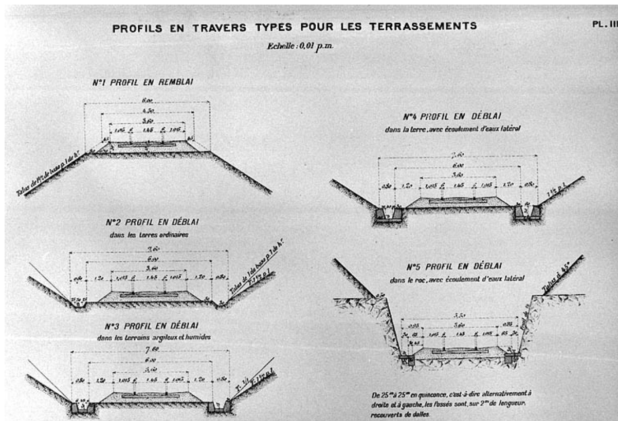
Profils en travers types pour les terrassements, [1919].
