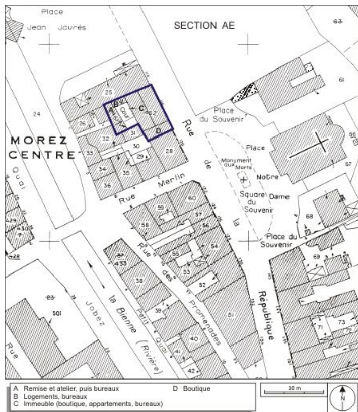
Plan-masse et de situation. Extrait du plan cadastral, 1980, section AI, échelle 1:1000. 39, Morez, 116 rue de la République
