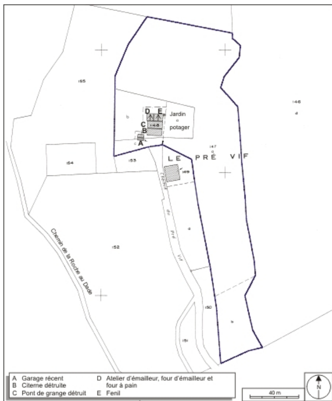
Plan-masse et de situation. Extrait du plan cadastral, 1980, section AE, échelle 1:1000 réduite à 1:1500. 39, Morez, 4 chemin du Pré vif, lieudit : le Pré vif
