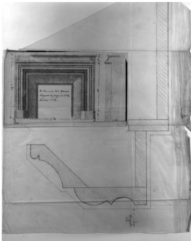
Production : projet de cheminée Louis XIII avec coupe d'un piédroit.
