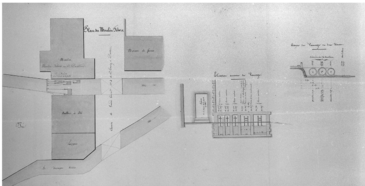
Réglementation des usines [...]. Plans et dessins de détail : détail du moulin Febvre.
