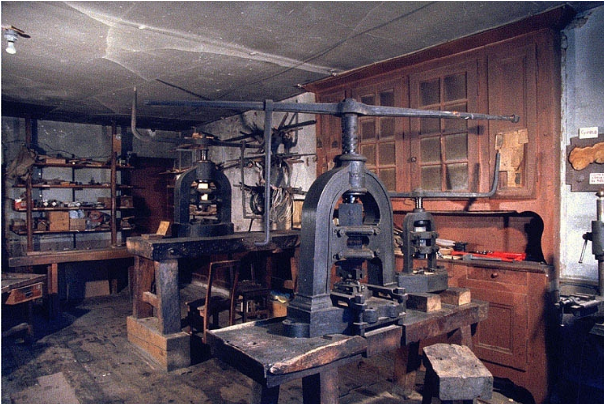
Presses à vis à balancier.
