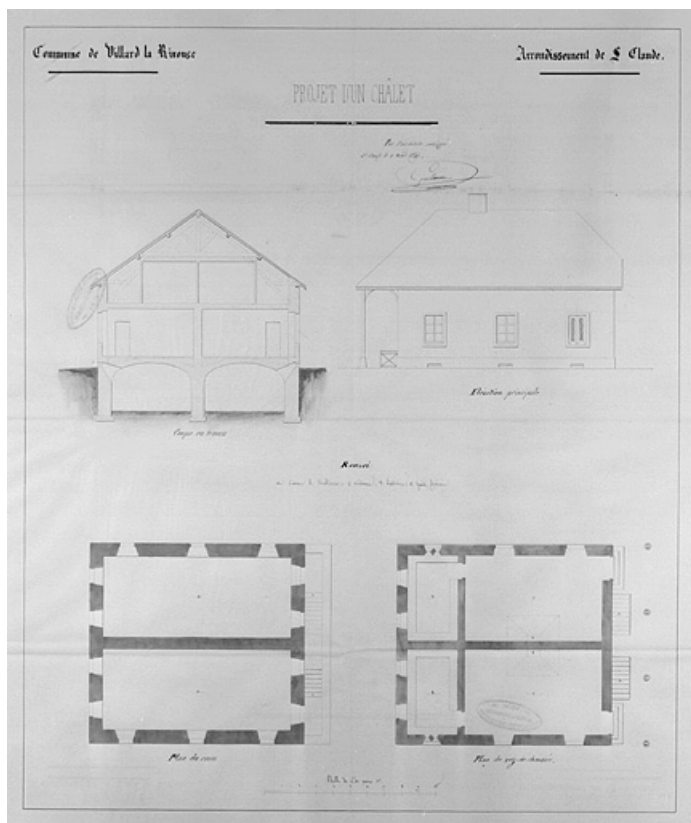
Projet d'un chalet : plan du rez-de-chaussée et des caves, façades, coupes. 39, Villard-sur-Bienne Vallée
