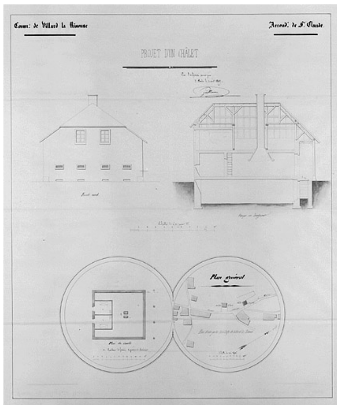
Projet d'un chalet : plan de situation, façade, coupe et plan des combles. 39, Villard-sur-Bienne Vallée
