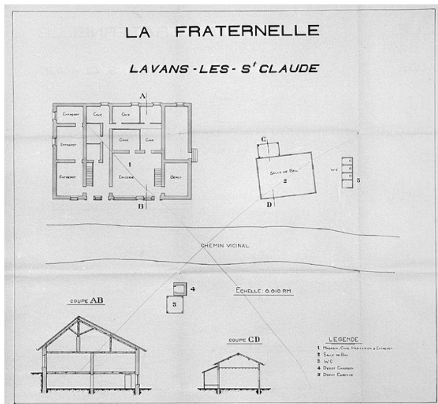
La Fraternelle. Lavans-lès-Saint-Claude [plan du rez-de-chaussée et coupe].
