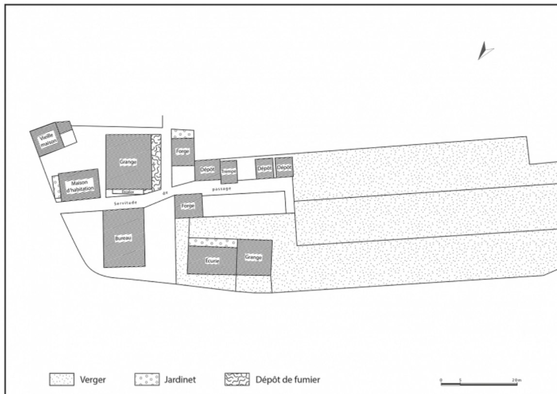
[Plan-masse et de situation avec affectation des bâtiments de Louis Gueutal Fils], 1916. 25, Montécheroux, 49-53 Grande Rue
