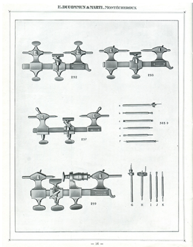
Tarif album n° 5. Fabrique d'outils E. Ducommun & Marti [catalogue de production, p. 56 : tours d'horloger et broches], [milieu 20e siècle].
