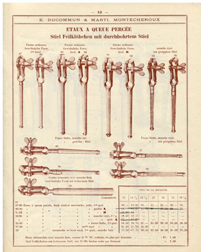
Tarif-album [...] E. Ducommun & Marti successeurs [catalogue de production, p. 13 : étaux], [années 1920-1930]. 25, Montécheroux, 1-3 rue de la Planchette
