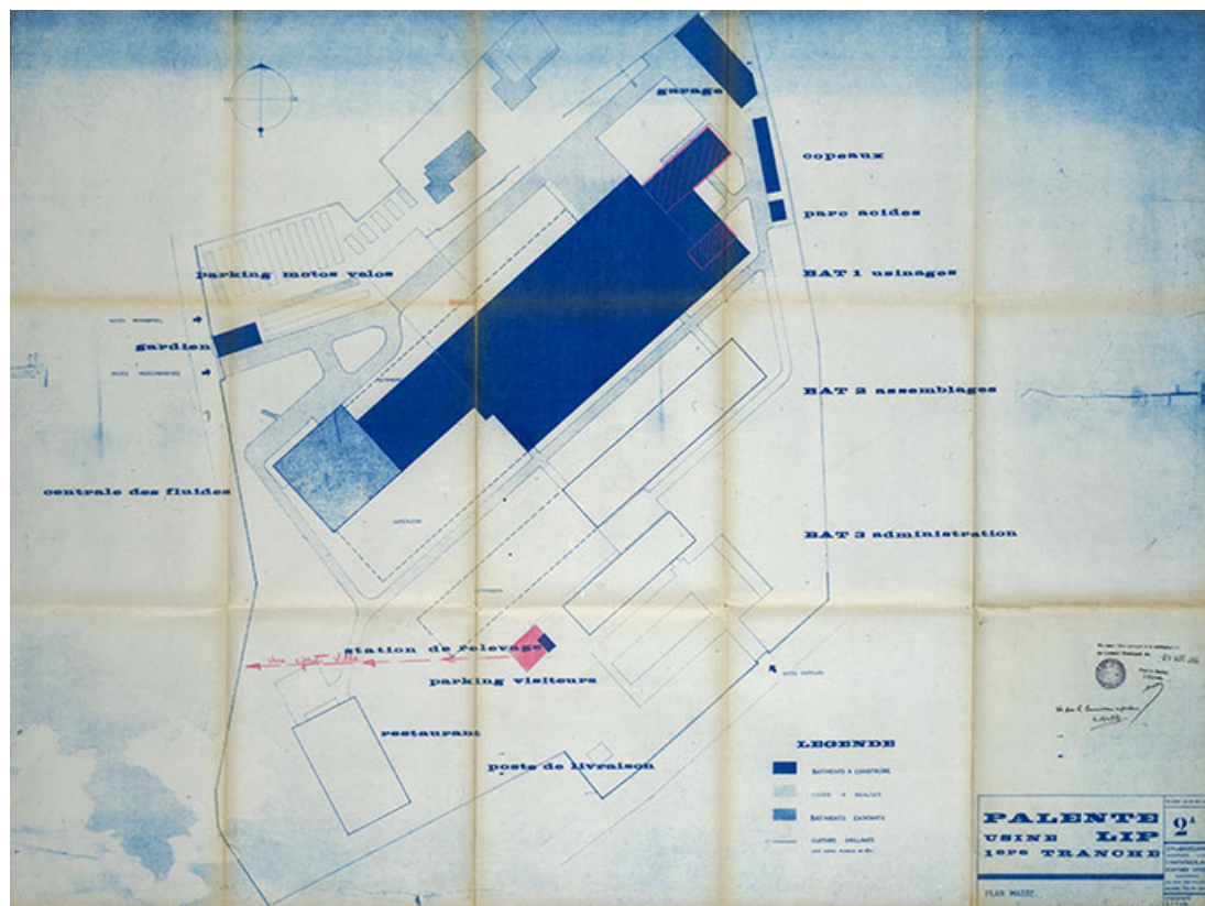
Usine Lip de Palente. Plan-masse, 1ère tranche (2A), 1959. 25, Besançon chemin de Palente
