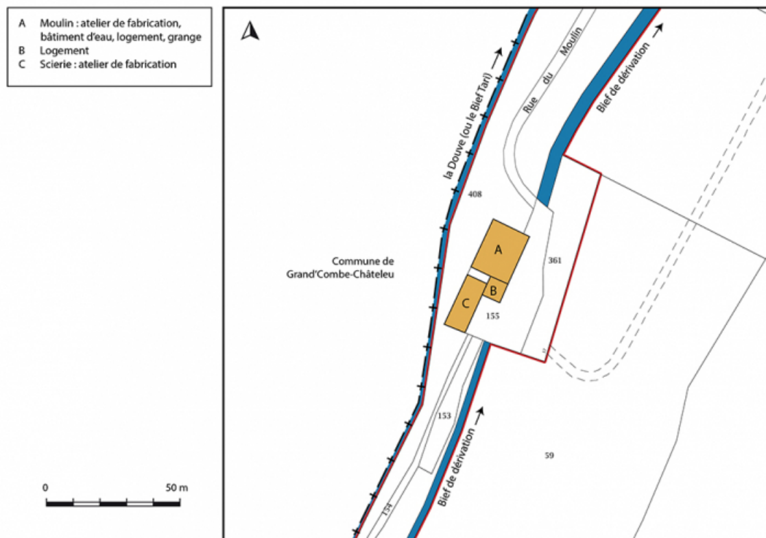
Plan-masse et de situation. Extrait du plan cadastral, 2016, section A, 1/2 500 agrandi à 1/1 000.
