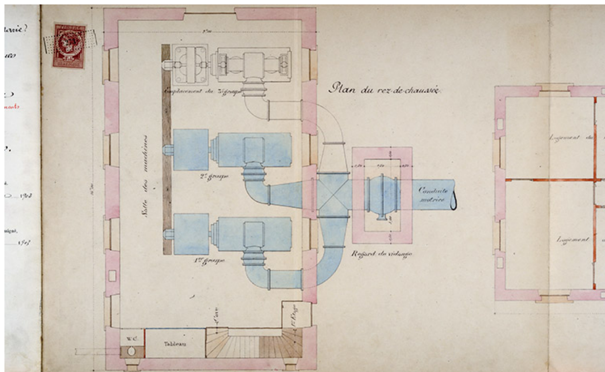
Projet d'exécution des ouvrages hydrauliques. Dessin du bâtiment [...]. Plan du rez-de-chaussée, 1903. 25, Labergement-Sainte-Marie, lieudit : le Fourpérét
