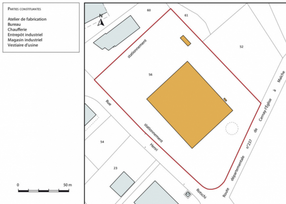
Plan-masse et de situation. Extrait du plan cadastral, 2015, section AM.
