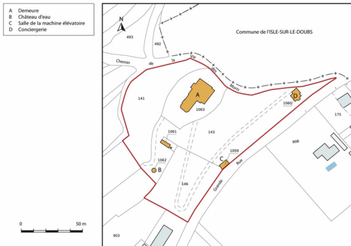
Plan-masse et de situation. Extrait du plan cadastral, 2015, section B. 25, Appenans route départementale 29
