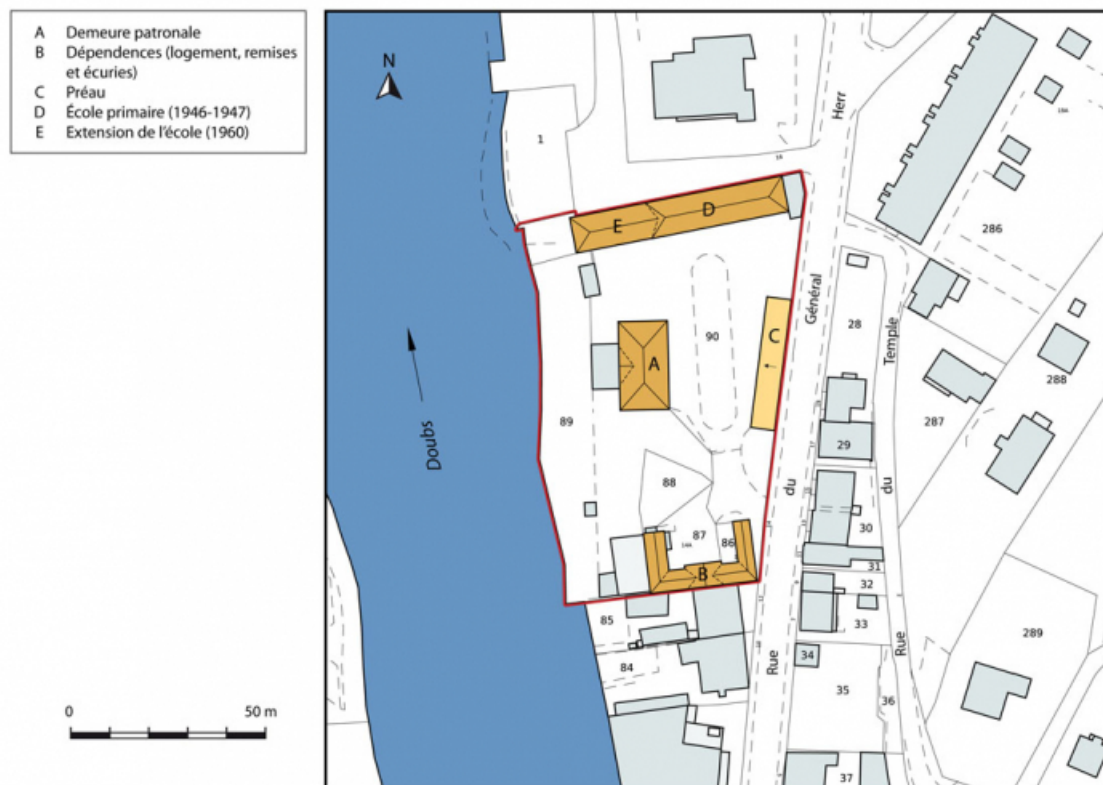
Plan-masse et de situation. Extrait du plan cadastral numérisé, section AO, échelle 1:1000.
