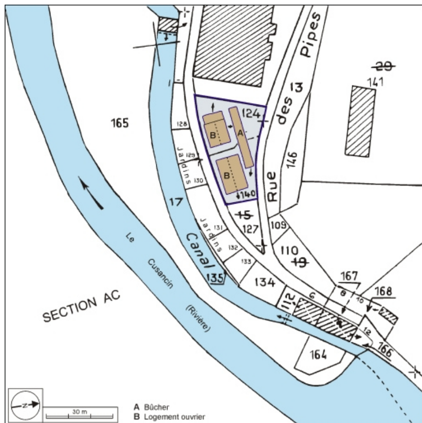
Plan-masse et de situation. Extrait du plan cadastral, 1982, section ZN, 1:2000 agrandi à 1:1000. 25, Baume-les-Dames, 9, 11 rue des Pipes, lieudit : Gondé
