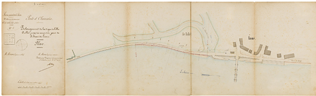
Plan du prolongement de la digue de l'île Rollet jusqu'en amont du pont de St Jean de Losne. 31 décembre 1852. 21, Losne
