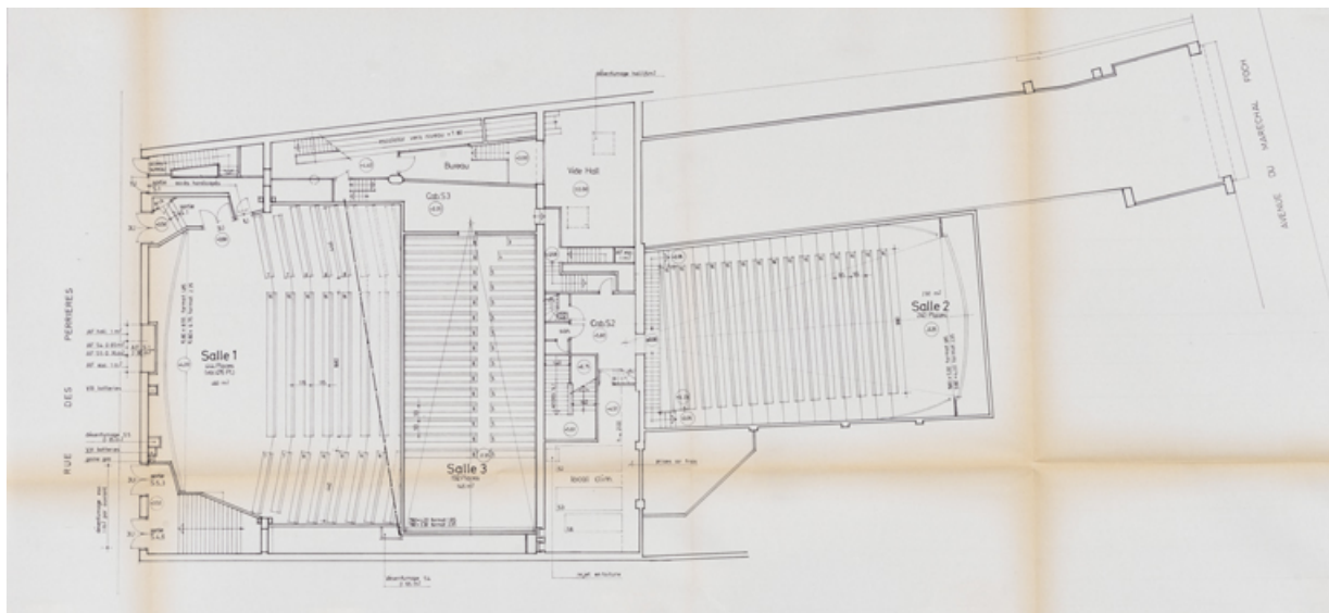
Cinémas Gaumont [...] Aménagement de 6 salles. Demande d'autorisation de travaux. Projet. 4. Plan du niveau rue des Perrières (+ 3.50 ; + 4.40). 18 avril 1990.
