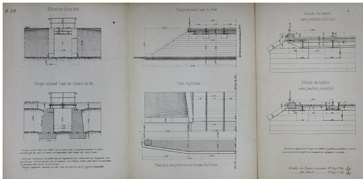
Pont sous rails à tablier métallique de 1 m 50 d'ouverture. Type de la Compagnie de Paris - Lyon - Méditerranée. E 29 [plan, coupes, élévation et détails], 1879.
