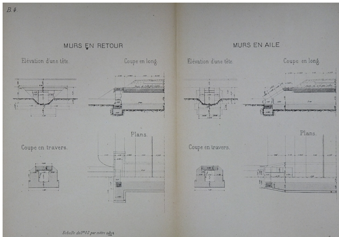
Aqueduc dallé de 0 m 60 d'ouverture. Type de la Compagnie Paris - Lyon - Méditerranée. B 4 [plans, coupes et élévations], 1879.
