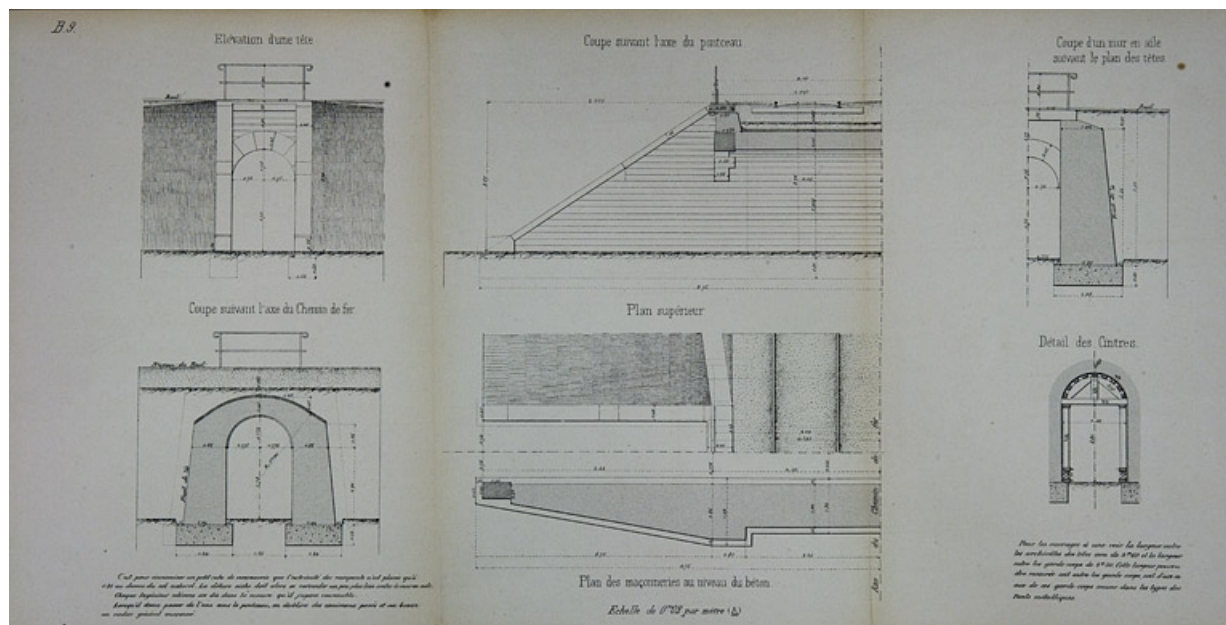
Aqueduc voûté de 1 m 50 d'ouverture. Type de la Comp[agn]ie de Paris - Lyon - Méditerranée. B 9 [plan, coupes et élévation], 1879.
