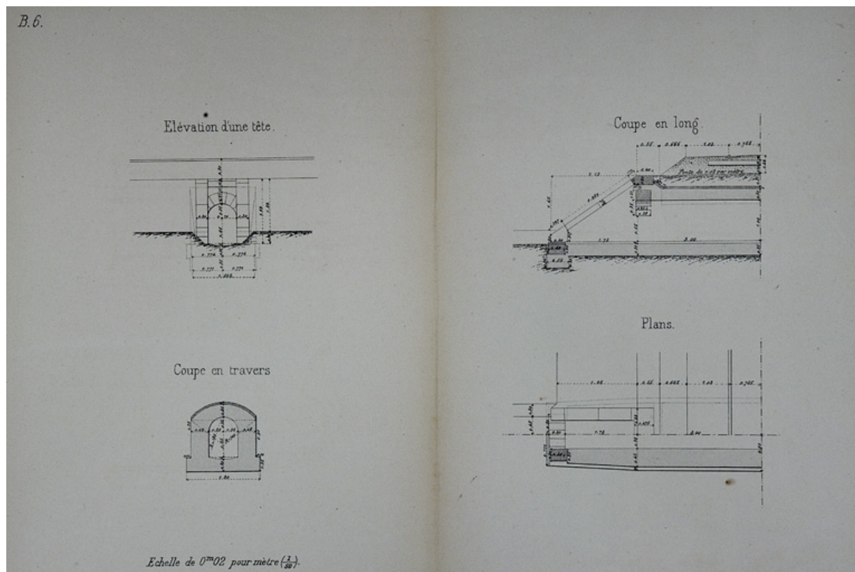
Aqueduc voûté de 0 m 70 d'ouverture. Type de la Compagnie de l'Est. B 6 [plans, coupes et élévation], 1879.
