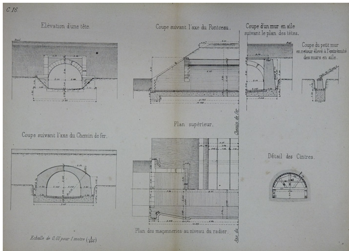
Pont sous rails de 4 m d'ouverture. Type de la Compagnie de Paris Lyon - Méditerranée. C 16 [plan, coupes et élévation], 1879.
