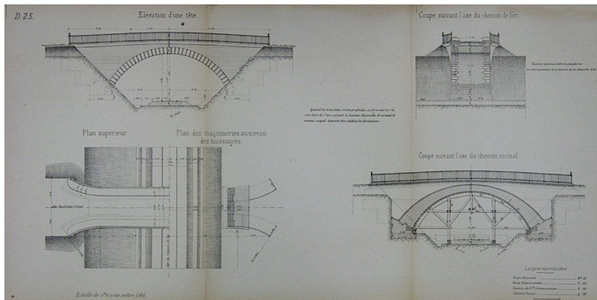
Pont sur rails à culées perdues de 12 m d'ouverture. Type de la Compagnie de Paris - Lyon - Méditerranée. D 25 [plan, coupes et élévation], 1879.
