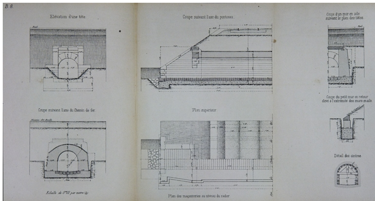
Aqueduc voûté de 1 m 50 d'ouverture. Type de la Cie Paris - Lyon Méditerranée. B 8 [plan, coupes et élévation], 1879.
