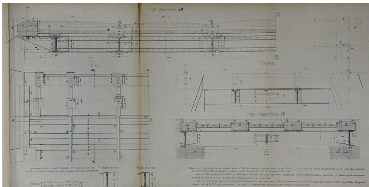
Pont sous rails à tablier métallique de 2 m d'ouverture. Type de la Compagnie de Paris - Lyon - Méditerranée. E 30 [détails du tablier : plan, coupes et élévation], 1879.
