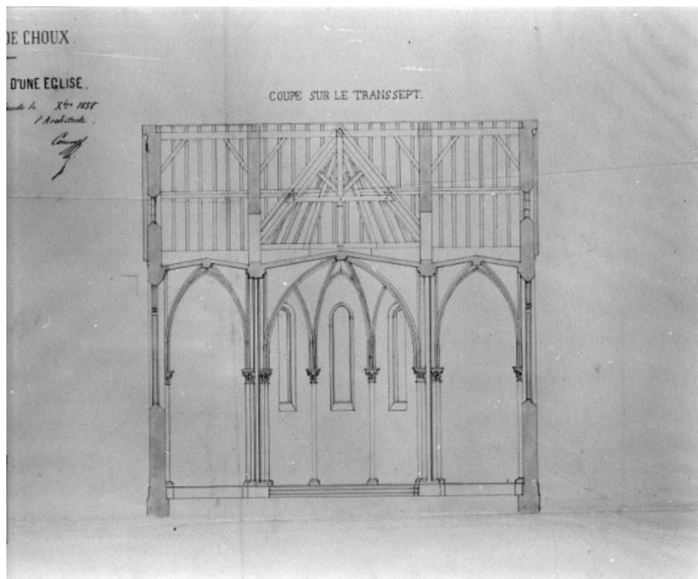
Commune de Choux. Construction d'une église [détail de la coupe sur le transept].
