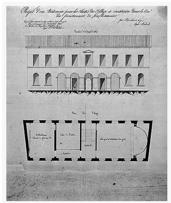
Plan et élévation du bâtiment annexe construit après 1828.
