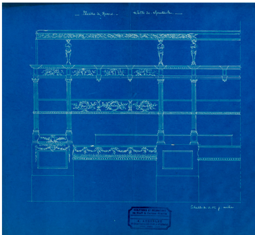
Théâtre de Nevers. Salle de spectacle [projet de décor, par Auberlet : élévation de la salle côté cour]. S.d. [1898]. 58, Nevers, 8 place des Reines de Pologne
