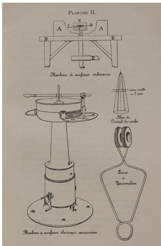
Machine à surfer ordinaire [et] Machine à surfer électrique américaine, 1913.
