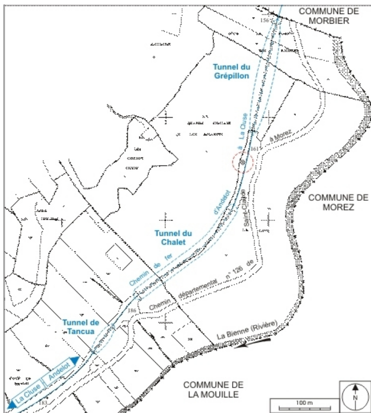
Plan de situation. Extrait du plan cadastral informatisé, 2006, section AD, échelle 1:4000. 39, Morbier, lieudit : la Côte
