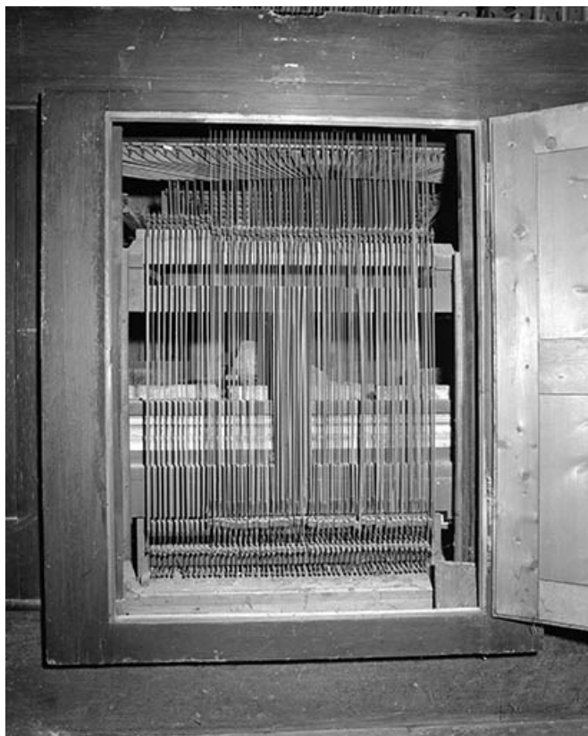
Mécanique : vergettes, vues de face.
