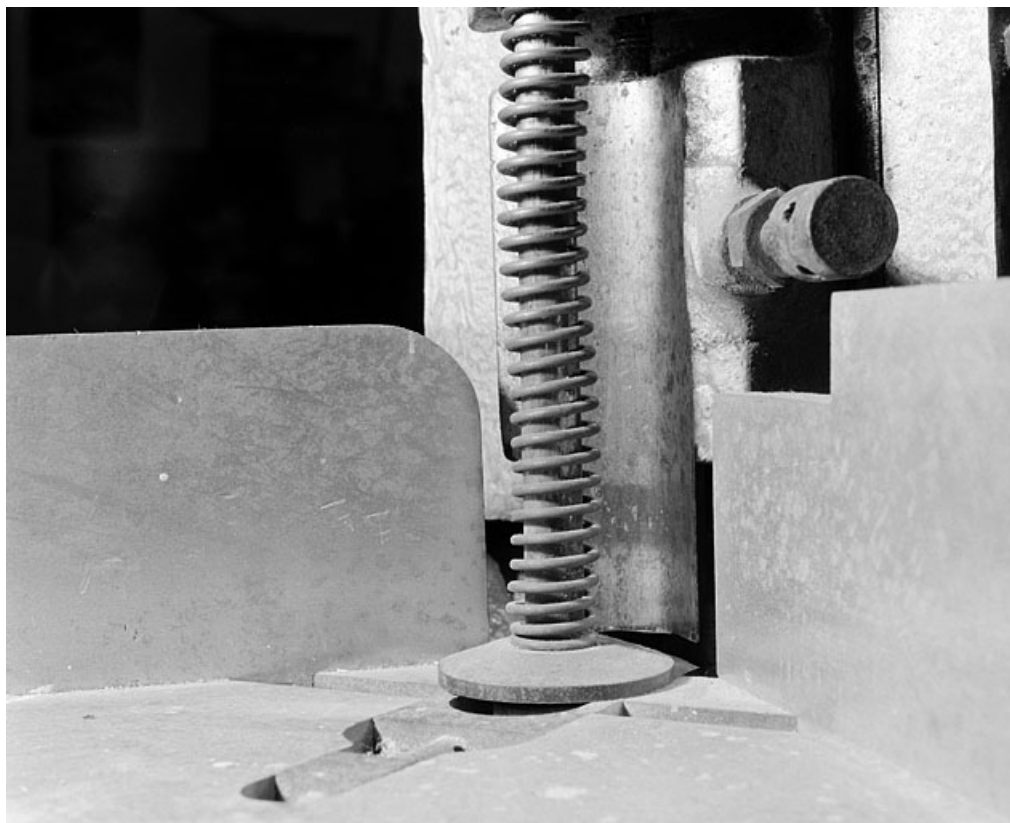
Détail du presse-papiers et du tranchoir.
