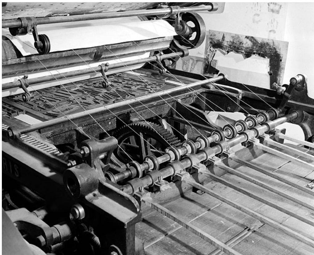
Partie arrière de la machine. Les fils permettent de soutenir la feuille qui sera déposée sur la table de réception, à droite, à l'aide du receveur mécanique à raquettes.
