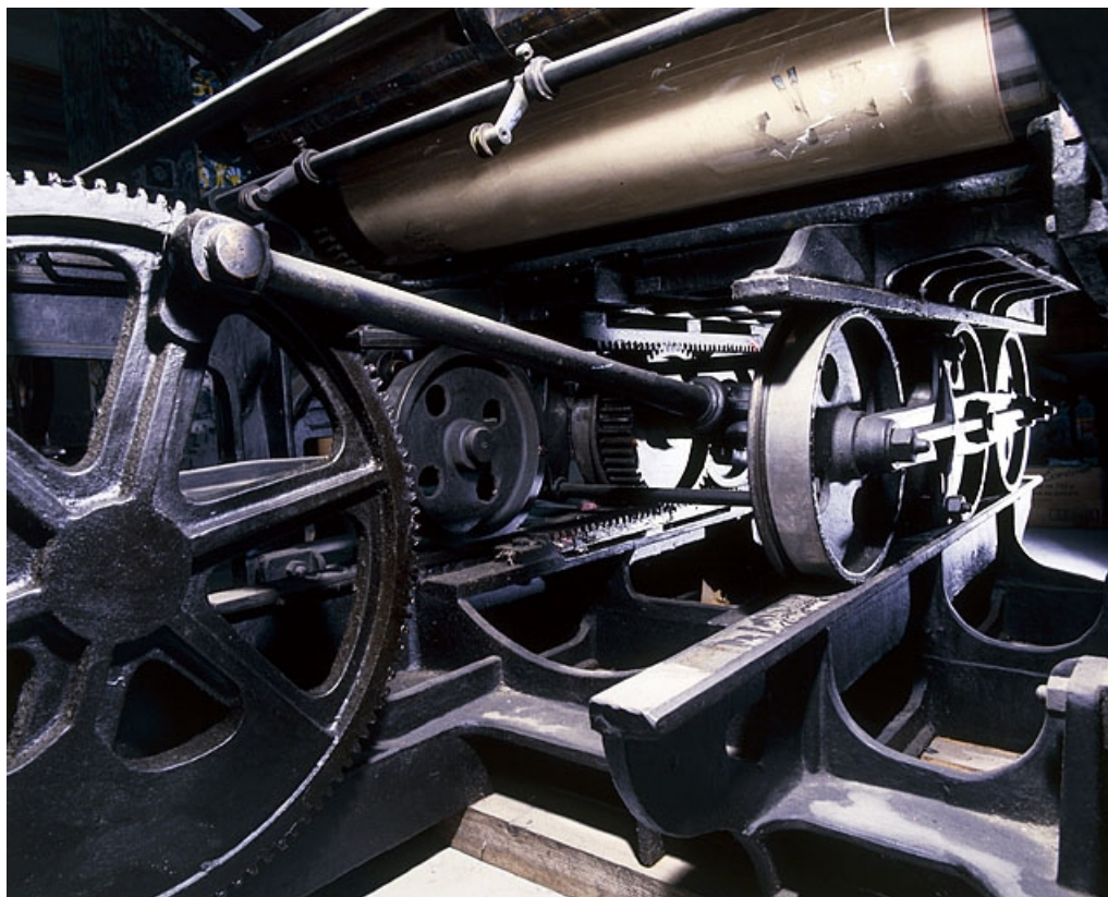
Système d'entraînement du marbre et son boggie. Le cylindre est visible en haut.
