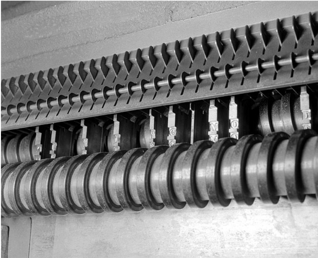
Vis d'entraînement et de distribution des matrices dans le magasin. En bas, extrémité des canaux du magasin. 39, Saint-Claude, 12 rue de la Poyat
