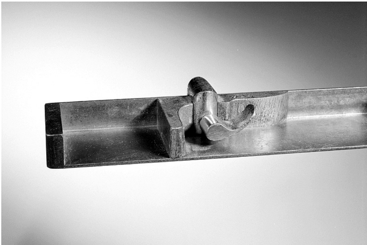
Blocage de l'équerre de l'un des compositeurs métalliques : système à levier à axe horizontal.
