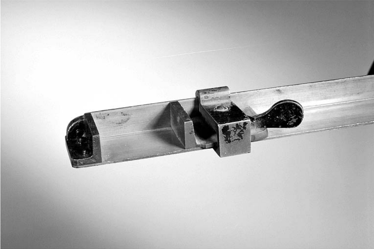
Blocage de l'équerre de l'un des compositeurs métalliques : système à levier à axe vertical.
