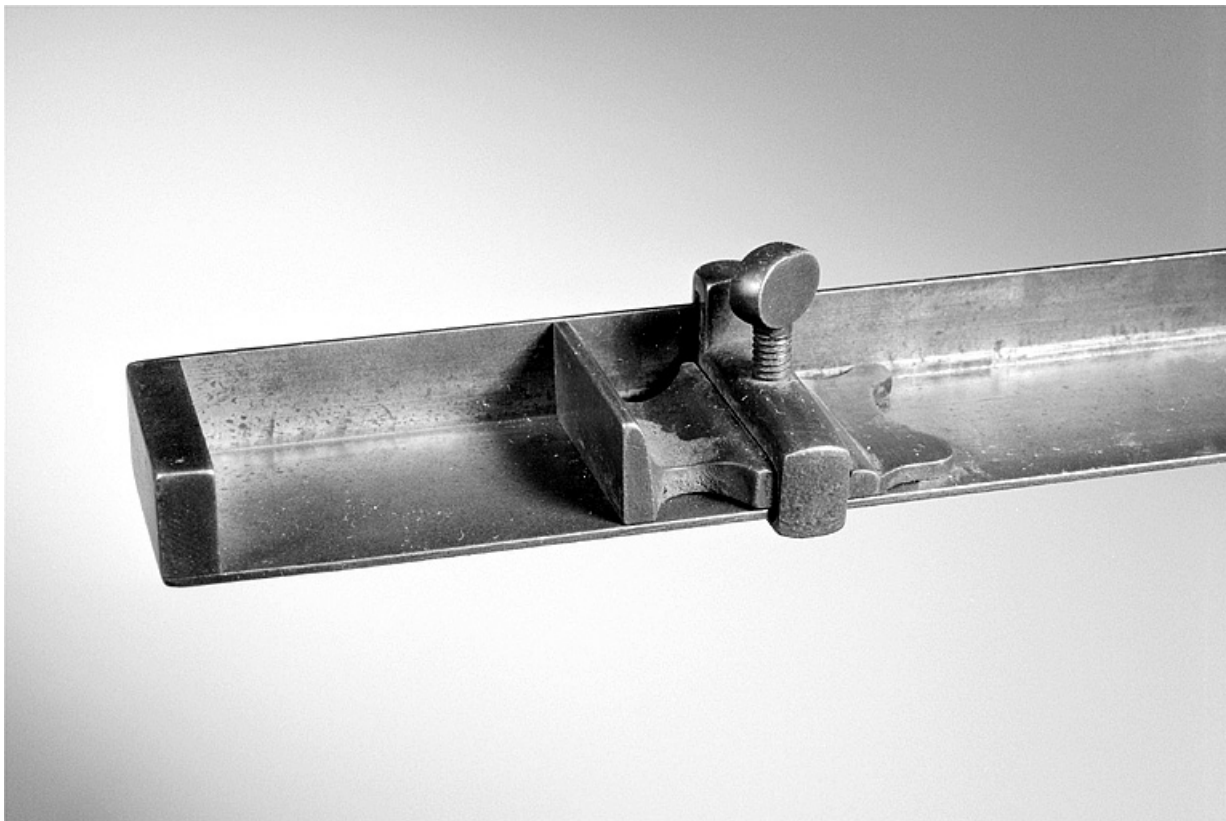
Blocage de l'équerre de l'un des compositeurs métalliques : système à vis.
