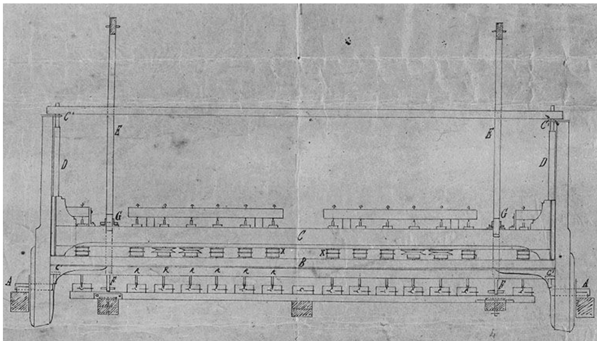
Elévation partielle de la face postérieure : détail du plan montrant le système d'entraînement des fraises et de fixation des ébauchons.
