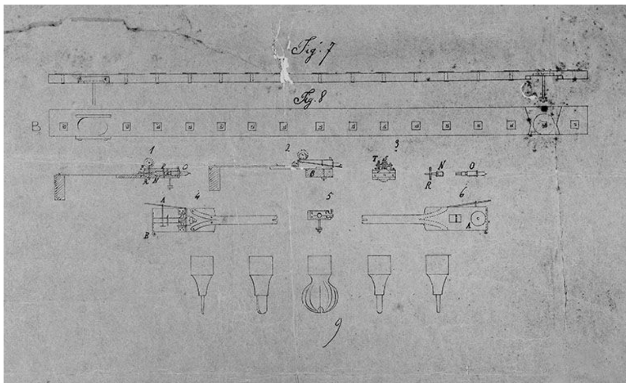
Dessins de détails : éléments du bâti, engrenages, système de rotation des supports d'ébauchons, fraises.
