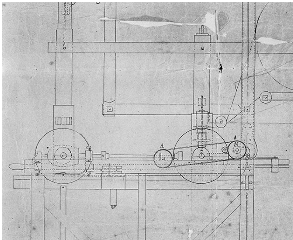
Élévation de la face latérale droite : détail de la partie centrale du plan.
