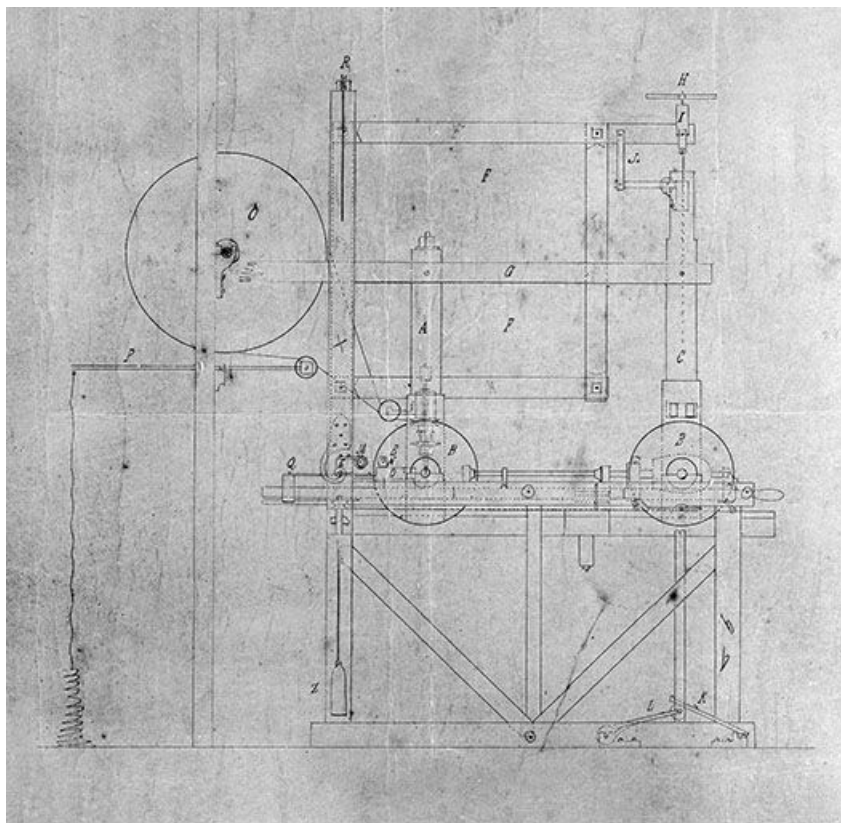
Elévation de la face latérale gauche.
