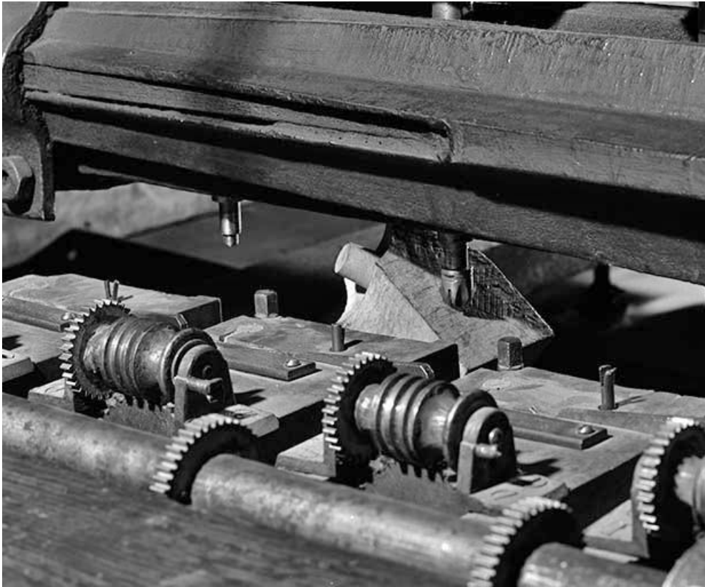
Face arrière : engrenages permettant la rotation simultanée des ébauchons (vue rapprochée). 39, Saint-Claude, 19 rue Carnot
