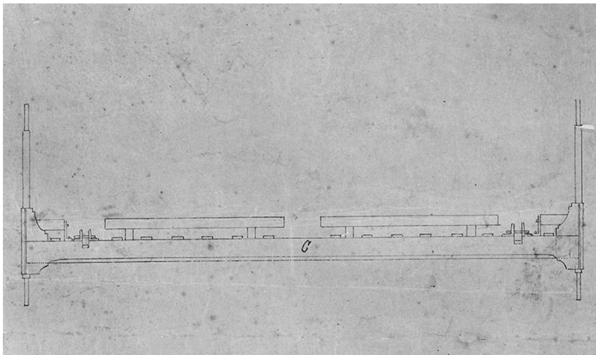
Elévation partielle de la face postérieure : détail du plan montrant une partie du bâti mobile.
