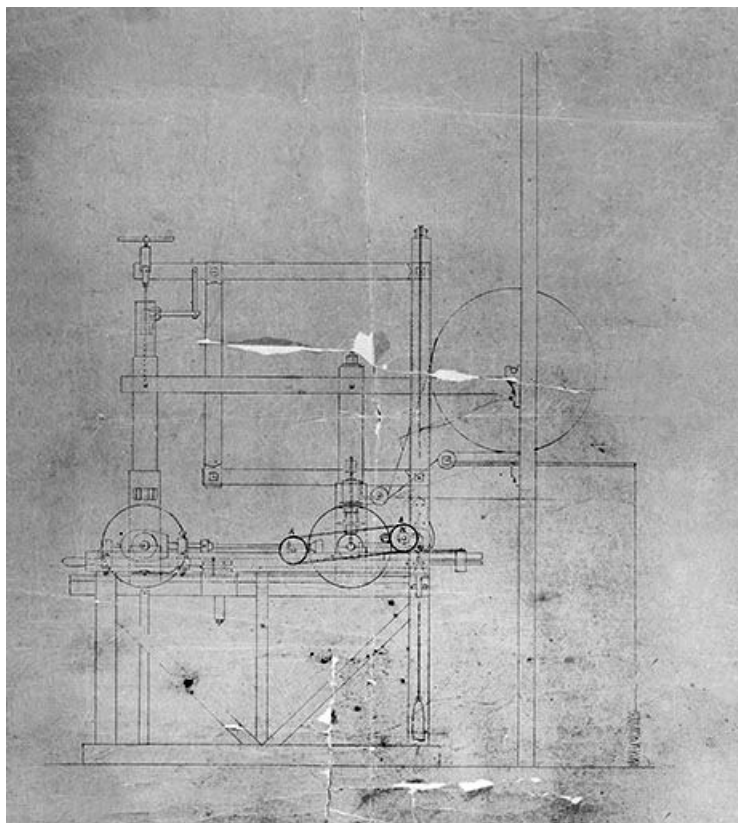
Elévation de la face latérale droite.
