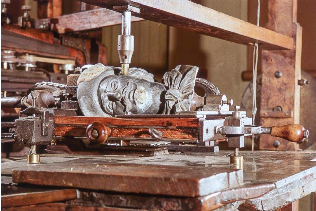
Modèle (d'Artagnan) et son support mobile, vus de trois quarts avant gauche. Manœuvré à l'aide des poignées, le support glisse sur une plaque métallique, chaque détail du modèle pouvant ainsi être retransmis par le palpeur vertical.
