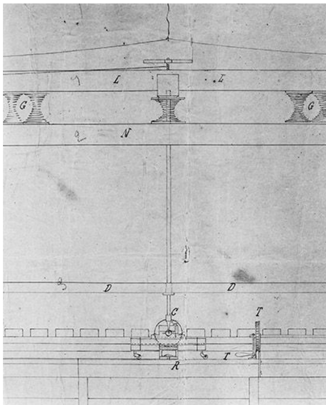
Elévation de la face antérieure : détail de la partie centrale du plan.
