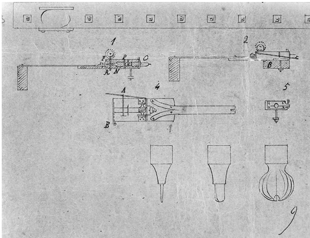
Dessins de détails [partie droite du plan] : éléments du bâti, engrenages, système de rotation des supports d'ébauchons, fraises. 39, Saint-Claude, 19 rue Carnot
