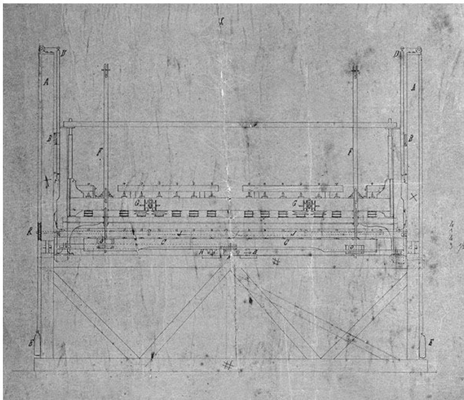
Élévation de la face postérieure.
