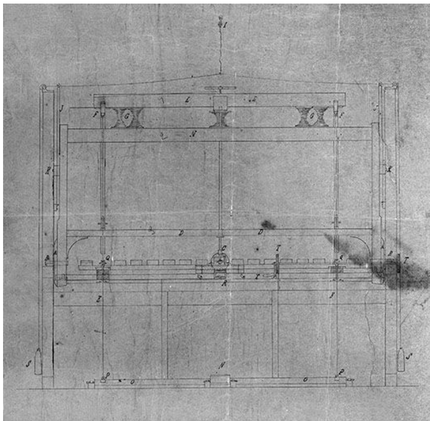
Elévation de la face antérieure.
