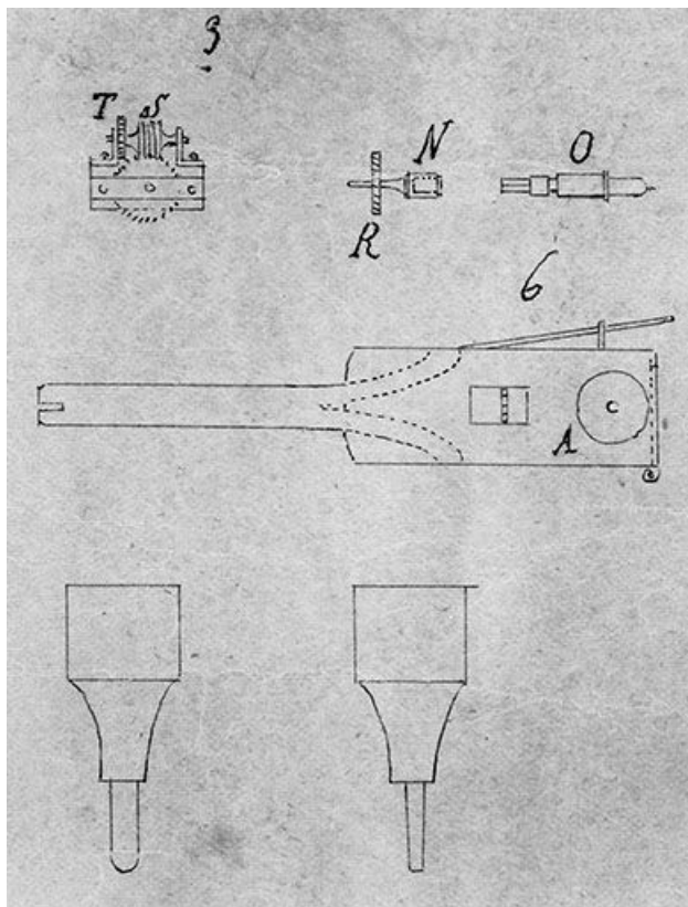
Dessins de détails [partie gauche du plan] : engrenages, système de rotation des supports d'ébauchons, fraises.
