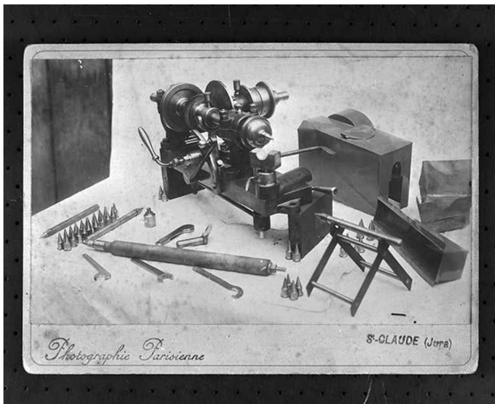
Exemple de machine à débiter du constructeur mécanicien Léon Lizon. 39, Saint-Claude
