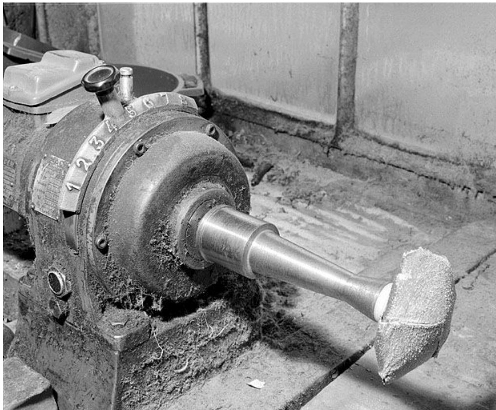
Vue rapprochée : variateur et disque de polissage.
