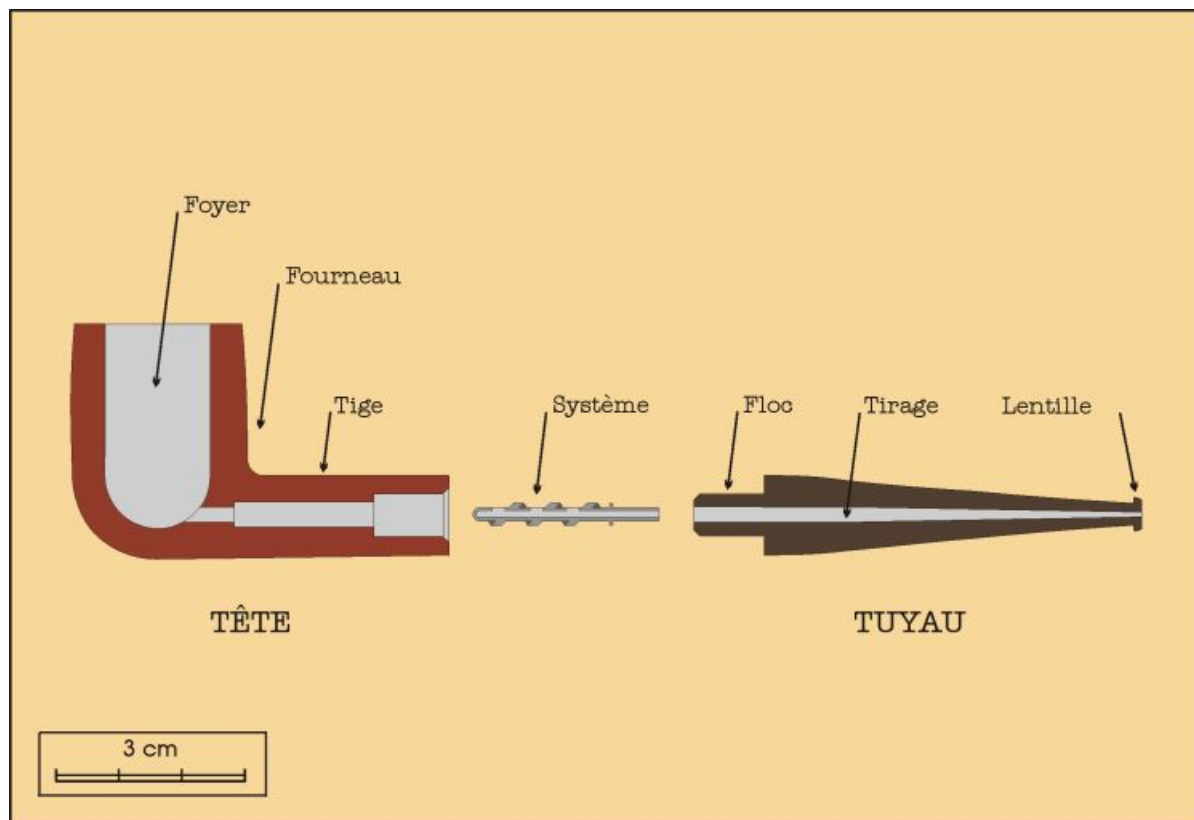
Coupe d'une pipe avec désignation de ses différentes parties.
