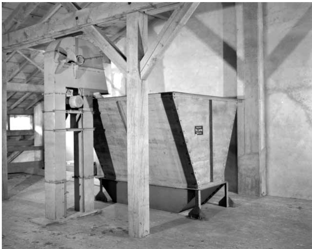
Module de chargement ou distributeur vibrant.
