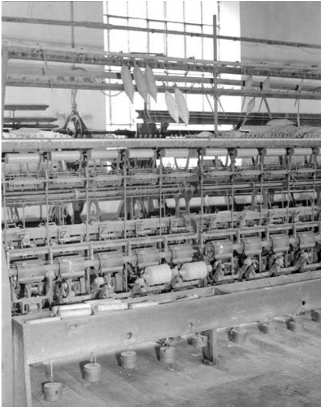
Détail d'une face vue de trois quarts, montrant 7 bobinois. De haut en bas, ratelier de dévidage à 2 niveaux supportant les bobines, tendeur, système de casse-fil, système de croisement des fils sur le bobinois, tambour moteur et bobinois.
