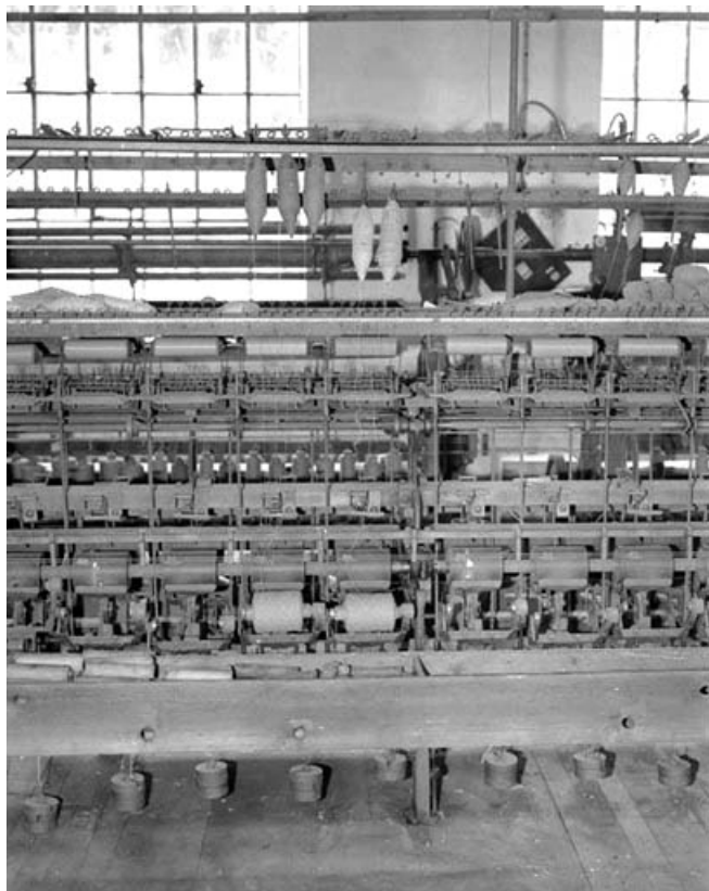
Détail d'une face, montrant 7 bobinots. De haut en bas, ratelier de dévidage à 2 niveaux supportant les bobines, tendeur, système de casse-fil, système de croisement des fils sur le bobinot, tambour moteur et bobinot.
