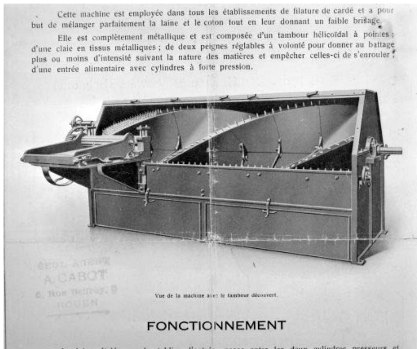
Vue de la machine avec le tambour découvert [exemple de batteur des Ets E. & J. Collette]. 39, Balanod, lieudit : sous Roches
