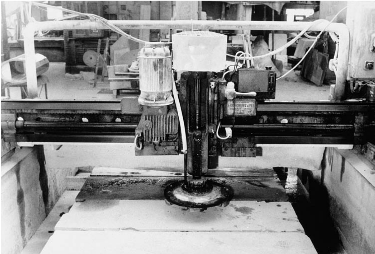
Polissoir est : bâti mobile et plateau de polissage.
